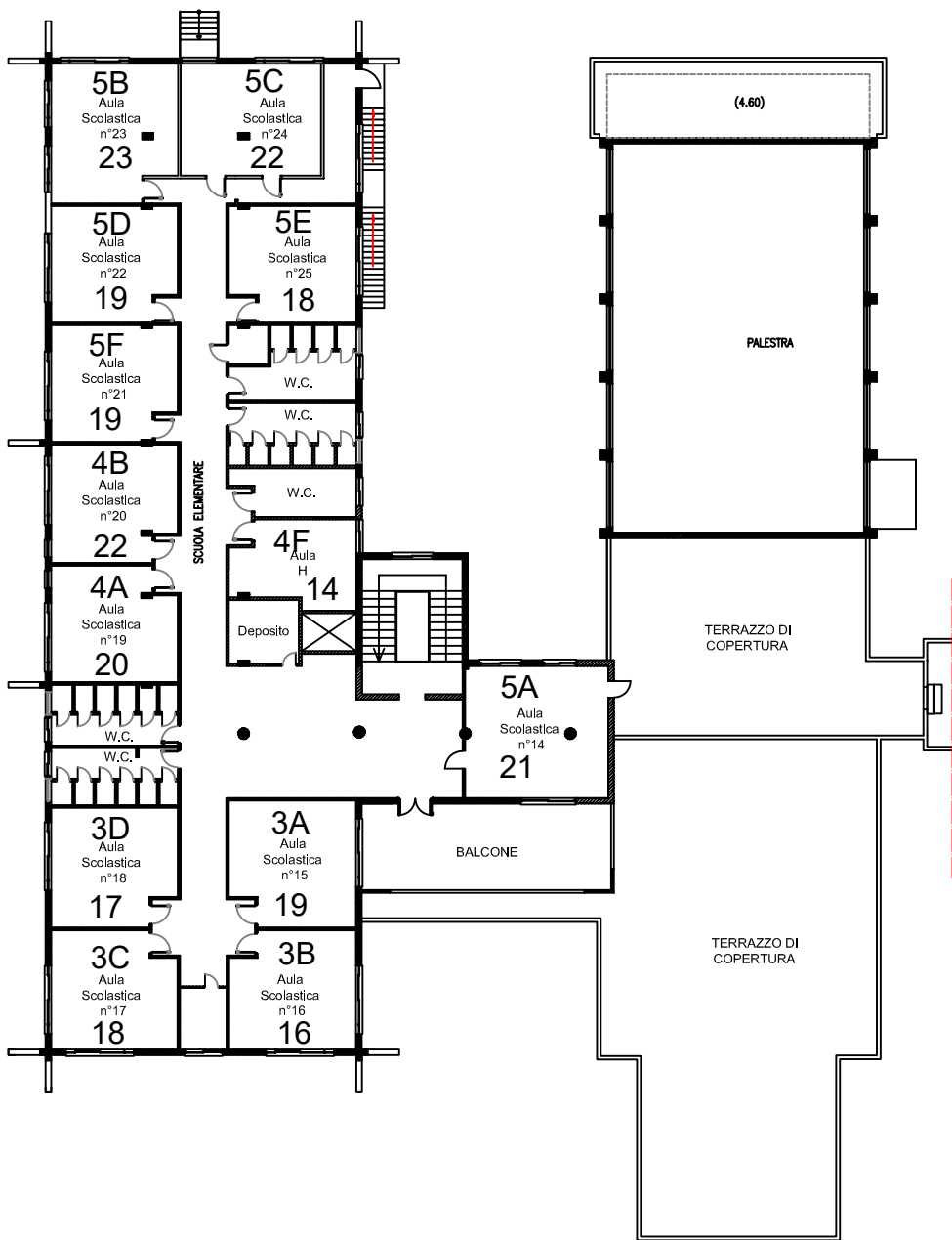
pianta piano primo – scala 1:200
